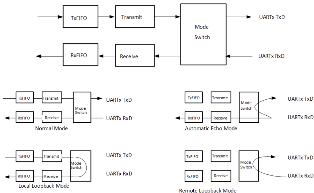
Figure: UART Mode Switch for Tx/D and Rx/D
