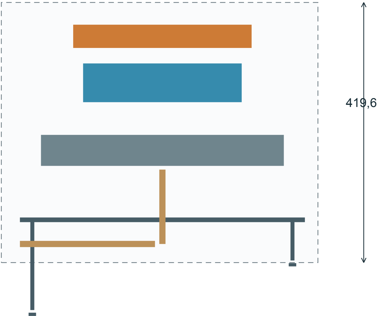
Вид сбоку: ось выходного вала Z = 400 Стойки до пола не входят в габарит ядра.
