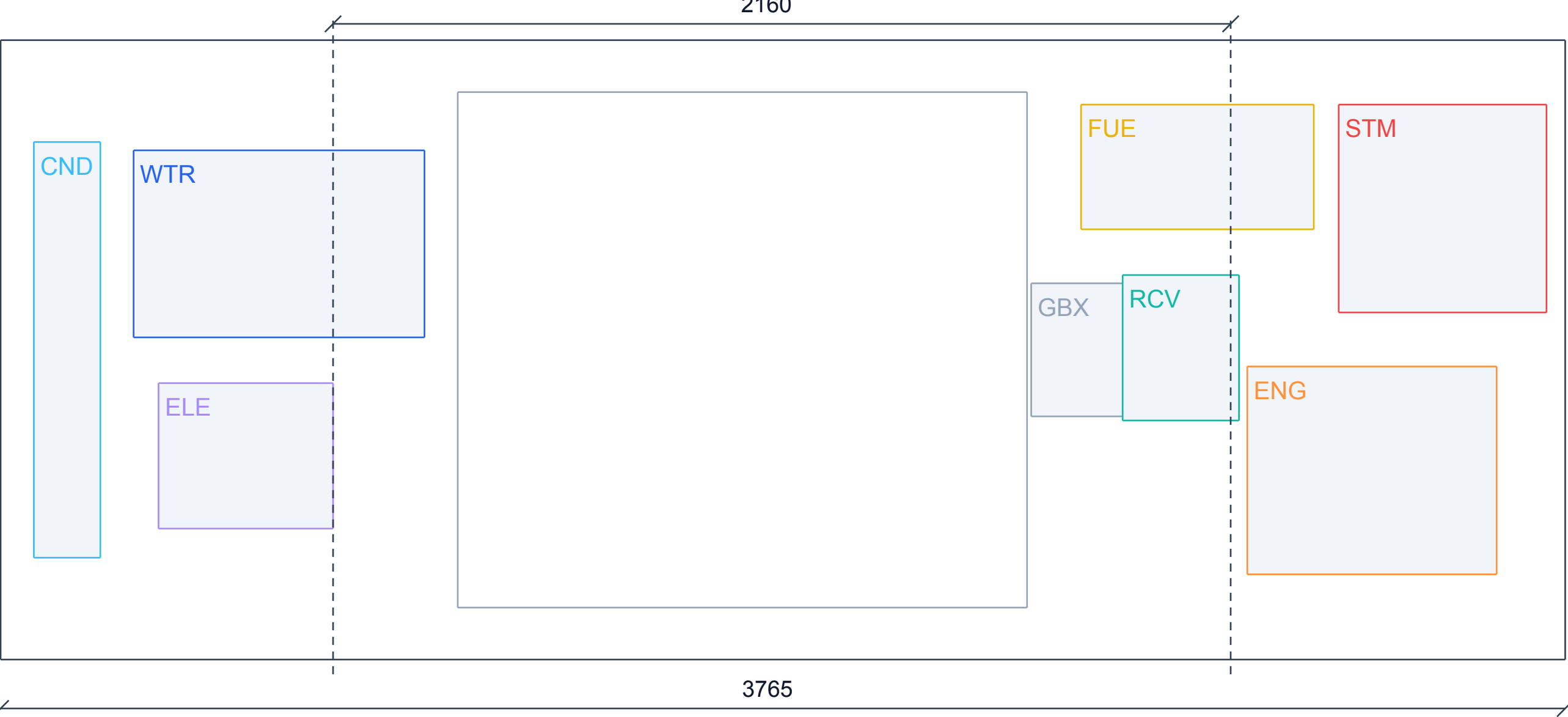
ВИД СВЕРХУ • перед автомобиля слева
