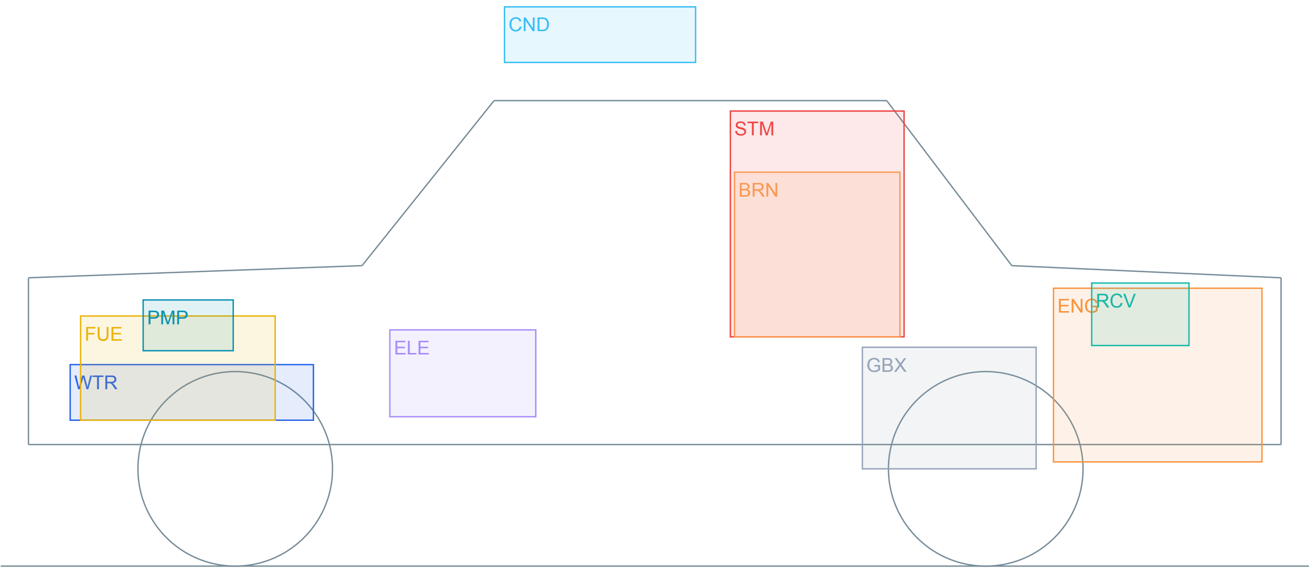
ВИД СБОКУ · разные высоты показывают разнесение агрегатов
