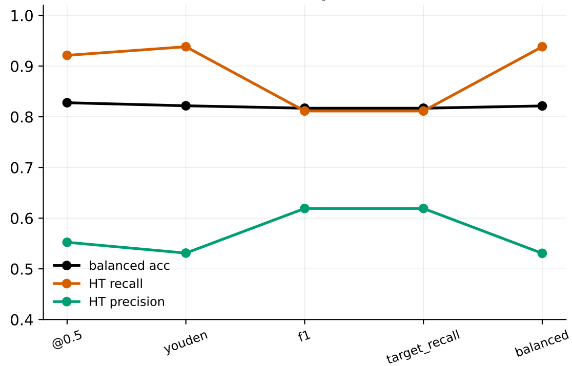
TabPFN · dependent
