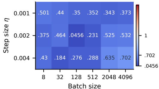
(d) ResNet-32 (no BN) \hat{H}
