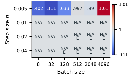
(d) ReLU MLP: 2 \times 512 \hat{H}
