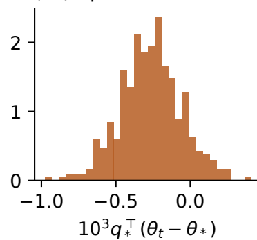
(d) Fixed-coordinate detail: updates 2048-2111
