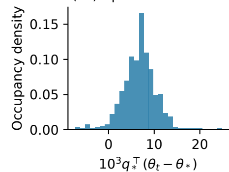
(c1) Updates 512-1023
