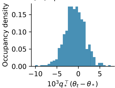
(c1) Updates 512-1023
