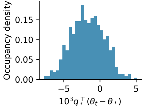
(c1) Updates 512-1023
