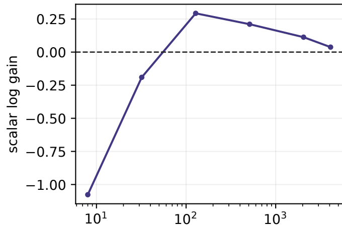
eta = 0.04
