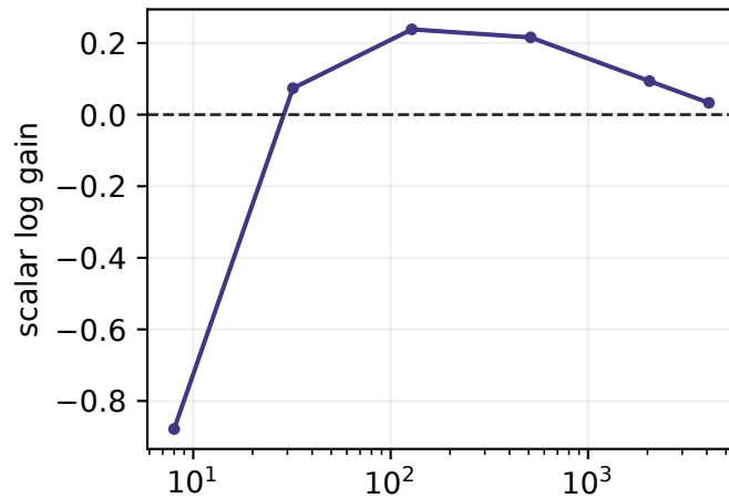
eta = 0.08
