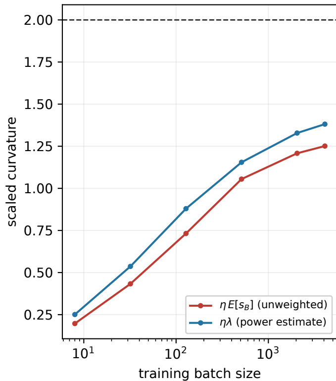
eta = 0.002 step 2,500
