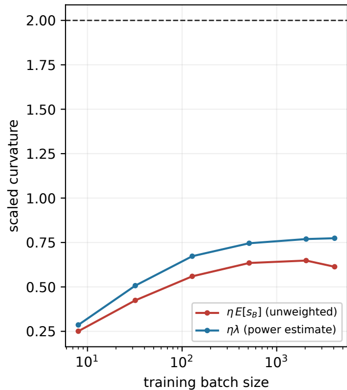
eta = 0.001 step 2,500
