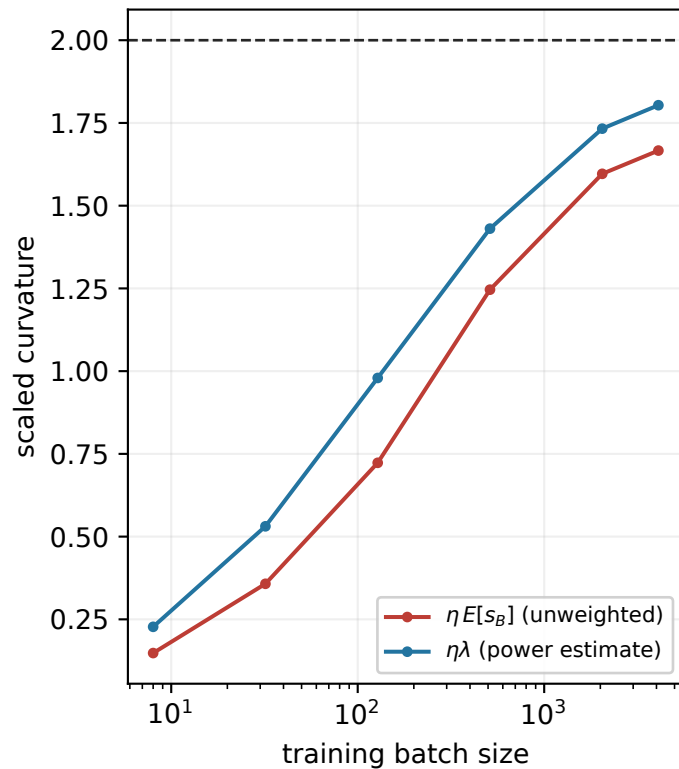
eta = 0.004 step 2,500
