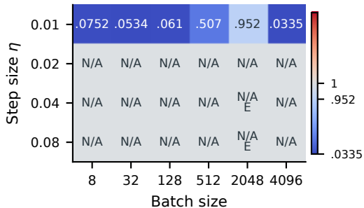
(d) ReLU MLP: 4 \times 512 \hat{H}
