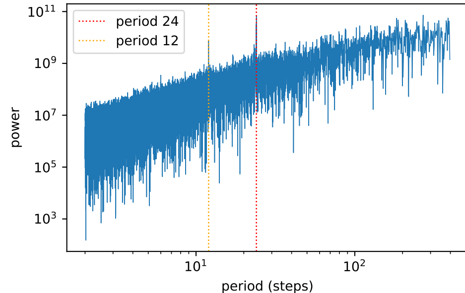
Periodogram (periods 2-400)
