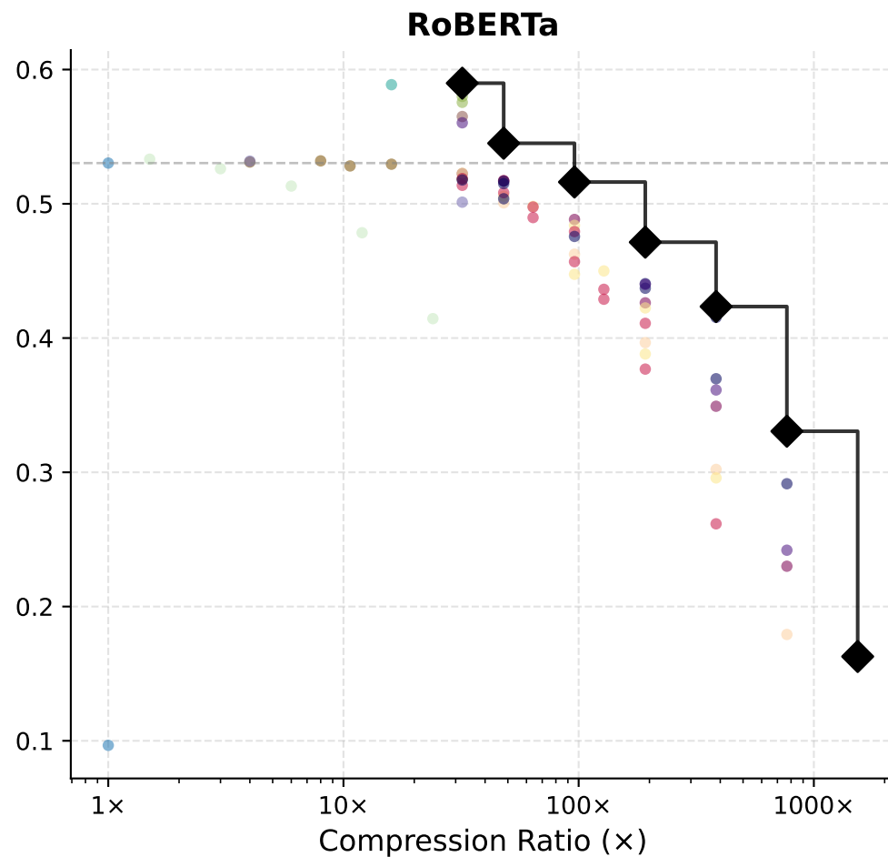
Pareto Frontier: MRR@10 vs Compression Ratio (all 224 variants)
