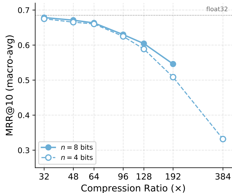
BGE
