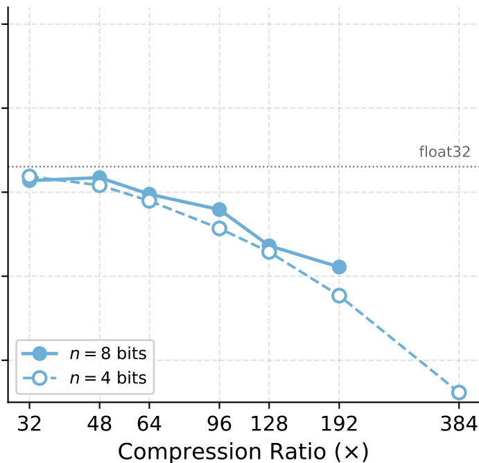
RoBERTa
