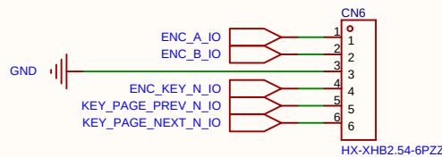
去交互板的接口
