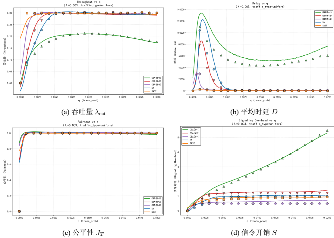
图 5-4 单节点到达率 \lambda = 0.003 ，流量类型为 uniform 场景下，AI 代理模型预测曲线（实线）与真实仿真结果（离散点）的性能对比。
