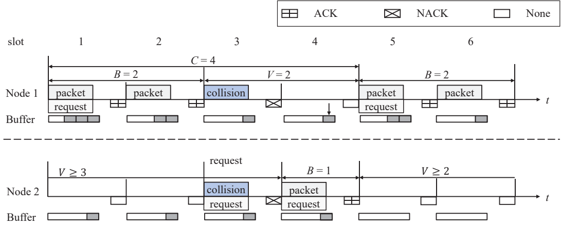
图 2-1 两节点 SAST 网络示意图，其中 B 、 V 和 C 分别表示节点的忙期、休假期和周期
