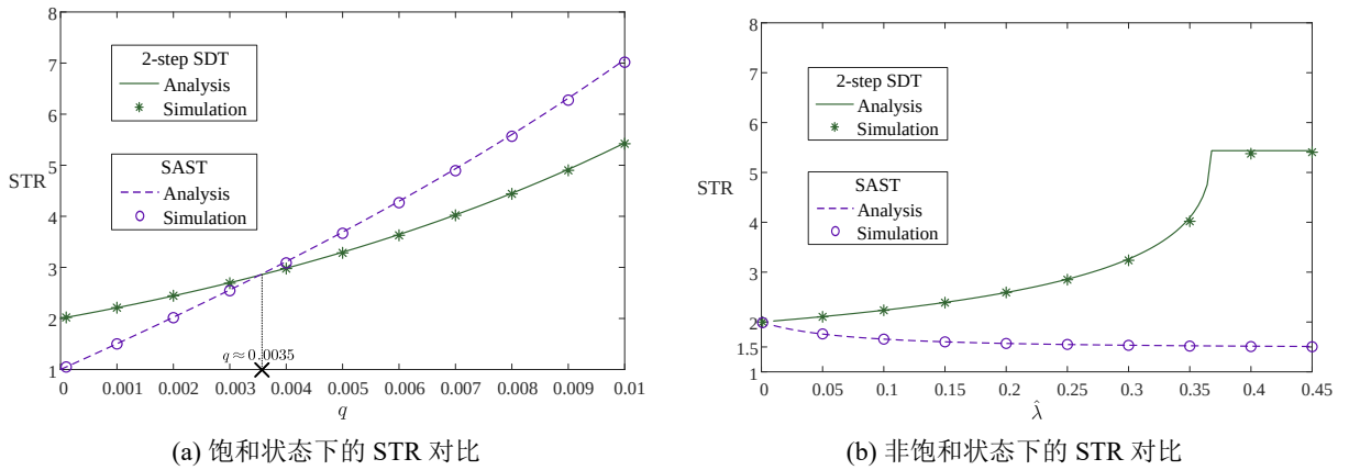
图 2-7 SAST 与 2-step SDT 方案的信令吞吐比 (STR) 性能对比 ( n = 100, s = 1 )
