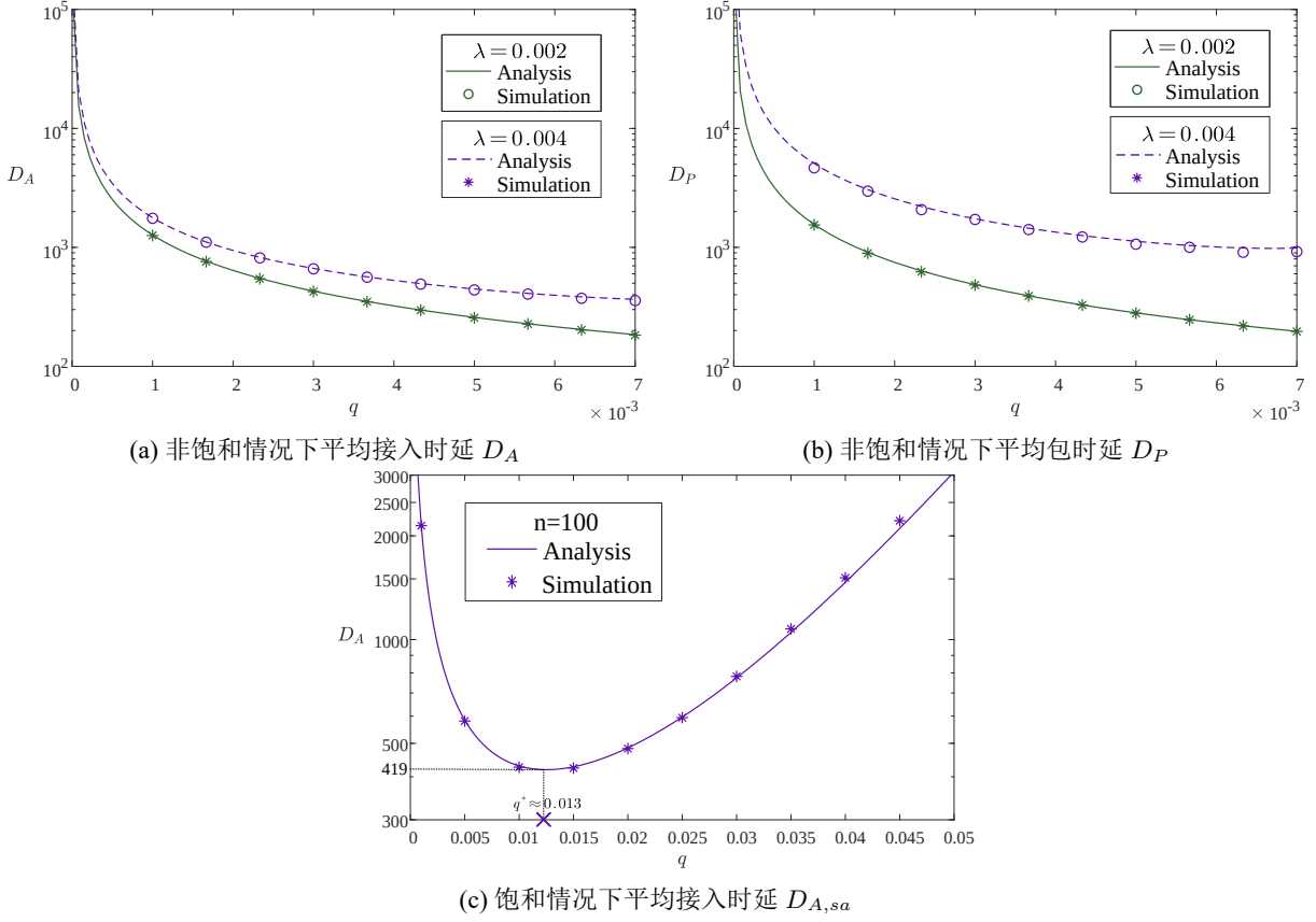
图 2-5 时延随传输概率 q 的变化情况 ( n = 100 , \lambda = \hat{\lambda}/n \in \{0.002, 0.004\} )
