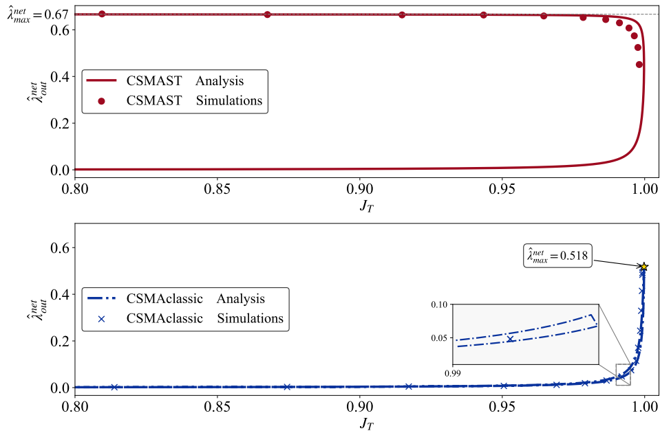
图 3-5 CSMAS 和经典 CSMA 方案下网络吞吐量 \hat{\lambda}_{out}^{net} 与短期 Jain 公平性指数 J_T 的关系。 n = 100 , q \in [0, 0.15] , \tau_F = x + 1 = 3 , \tau_I = 1 , \tau_S = y + 1 = 5 , T = 10^6 个时隙。
