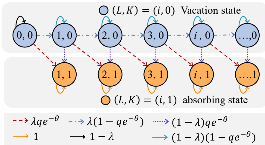
图 4-2 描述忙期内队列演化的吸收马尔可夫链状态转移图
