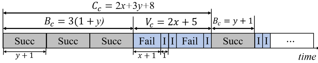
图 3-1 CSMAST 方案中的信道示意图, 其中 B_c 、 V_c 和 C_c 分别表示信道的忙期、休假期和周期时间。符号“Succ”、“Fail”和“I”分别表示三种基本信道状态: 成功传输、碰撞和空闲。
