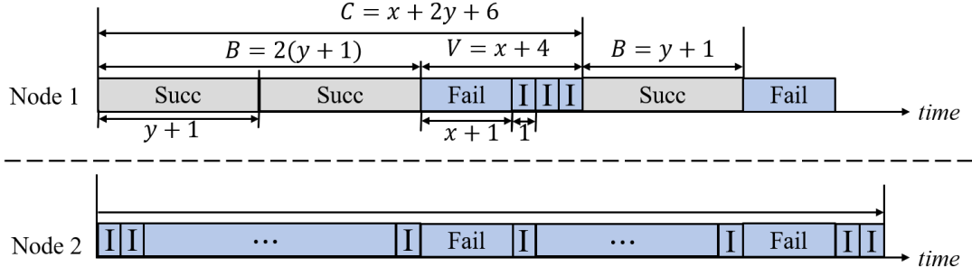
图 3-2 两个 CSMA/ST 节点之间的时间交互示意图，其中 B 、 V 和 C 分别表示节点的忙期、休假期和周期时间。
