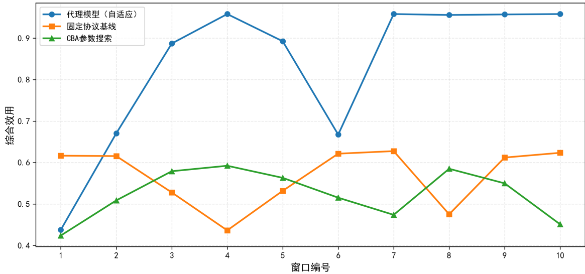
图 5-6 动态业务场景下代理模型推荐策略与基线策略的效用对比。横坐标表示按时序排列的协议切换窗口编号，纵坐标表示对应的综合效用 U(\bar{y}) 。
