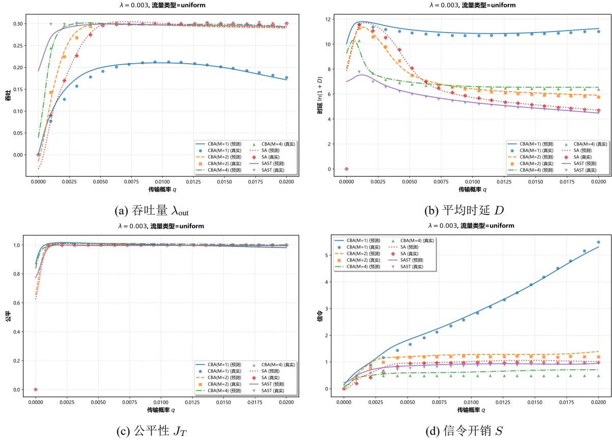
图 5-4 单节点到达率 \lambda = 0.003 、uniform 流量场景下，代理模型预测曲线（实线）与仿真结果（离散点）的性能对比。
