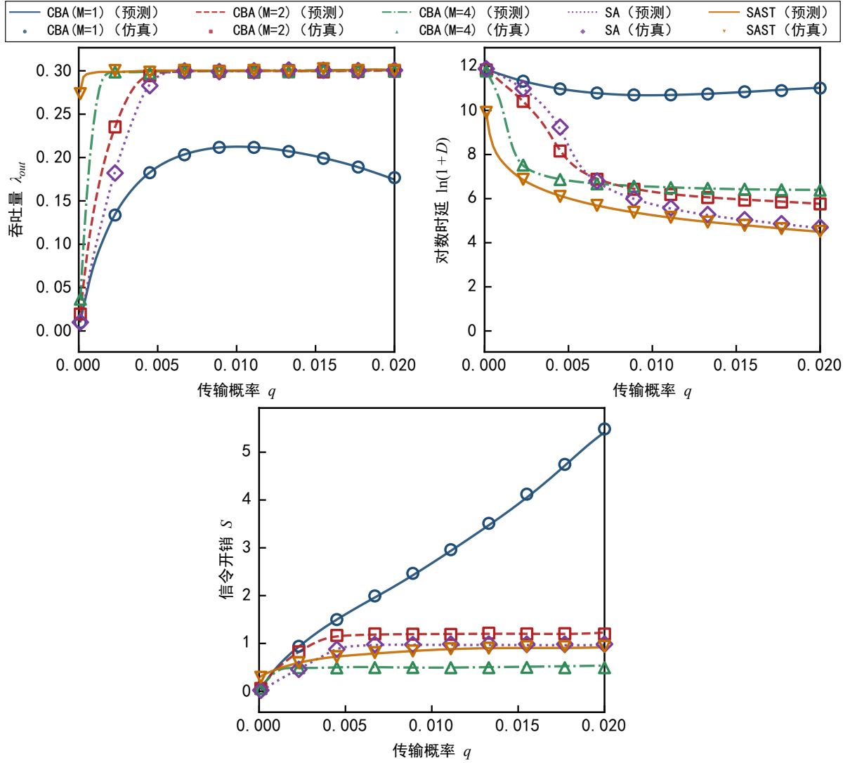
图 5-5 均匀流量、 \lambda = 0.003 场景下的模型预测数值与仿真结果对比。
