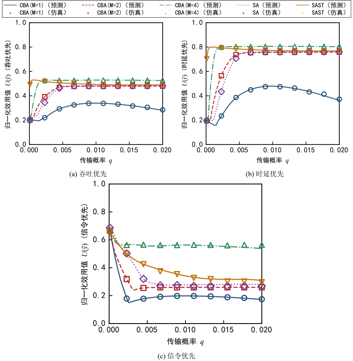
图 5-6 均匀流量、 \hat{\lambda} = 0.003 场景下，不同权重偏好的综合效用 U 对比。
