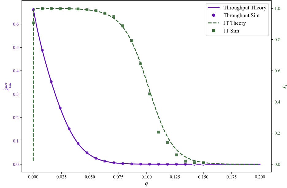
图 4-3 CSMAS 网络吞吐量 \hat{\lambda}_{out}^{net} 与短期 Jain 公平性指数 J_T 随传输概率 q 的变化 ( n = 100, \tau_S = 5, \tau_F = 3, \tau_I = 1, T = 10^6 )
