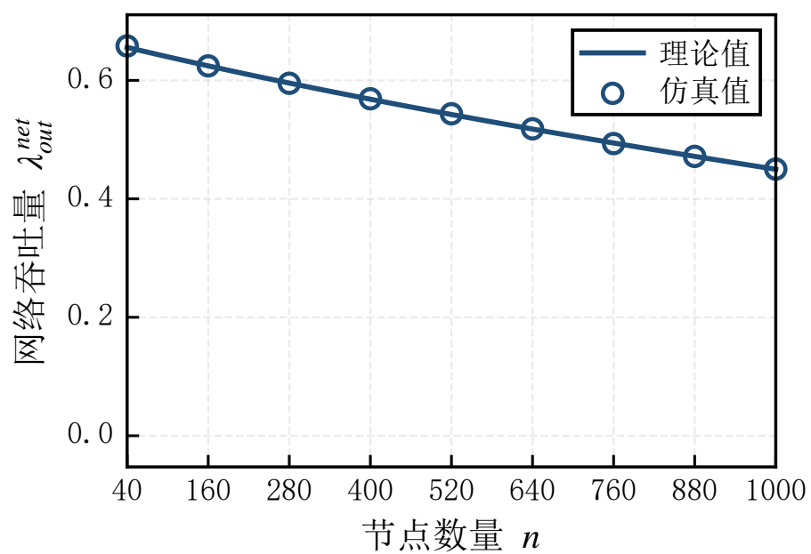
图 4-4 CSMAST 网络吞吐量 \lambda_{out}^{net} 随节点数量 n 的变化（理论值与仿真值对比）
