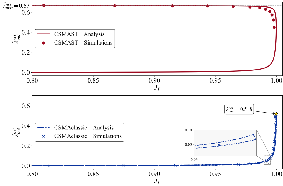
图 4-5 CSMAST 与经典 CSMA 方案的吞吐量-公平性性能轨迹对比
