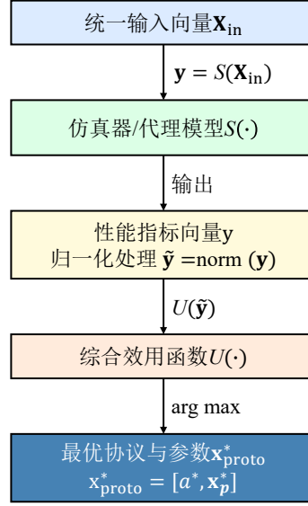
图 5-1 统一接入框架与协议选择流程
