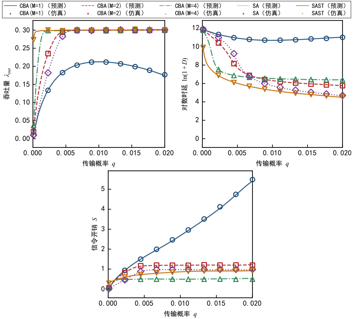
图 5-5 均匀流量、归一化总到达率 \lambda = 0.3 场景下的模型预测数值与仿真结果对比。节点数量为 n = 100 。时隙总长度为 t = 10^6 。
