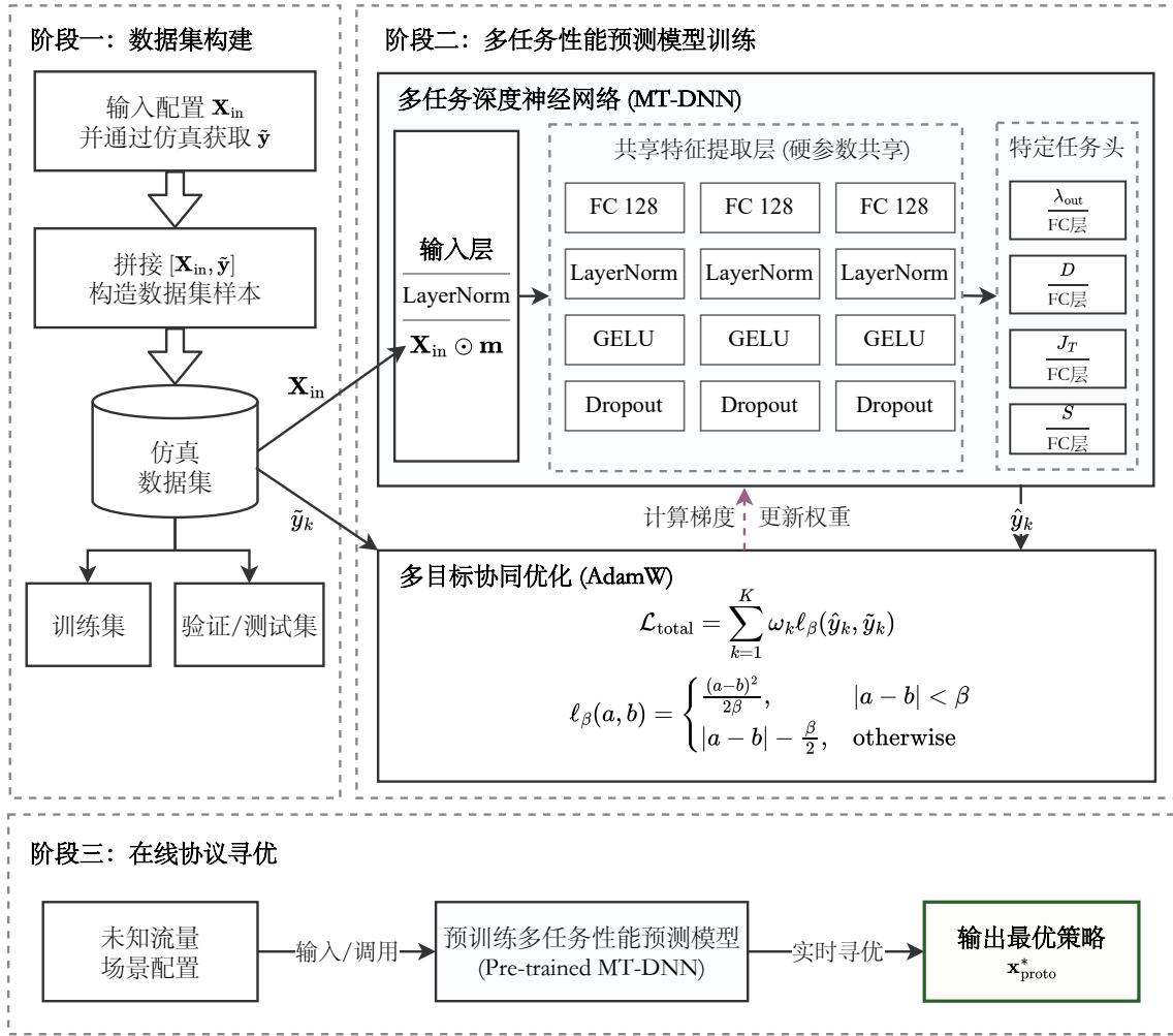
图 5-4 多任务性能预测模型的训练流程示意图
