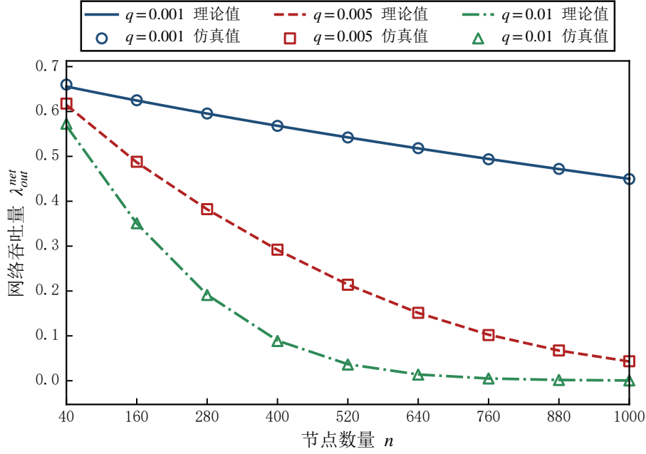
图 4-5 CSMAST 网络中 \lambda_{out}^{net} 随节点数量 n 的变化（多组 q 叠加， \tau_S = 5, \tau_F = 3, \tau_I = 1, T = 10^6 ）
