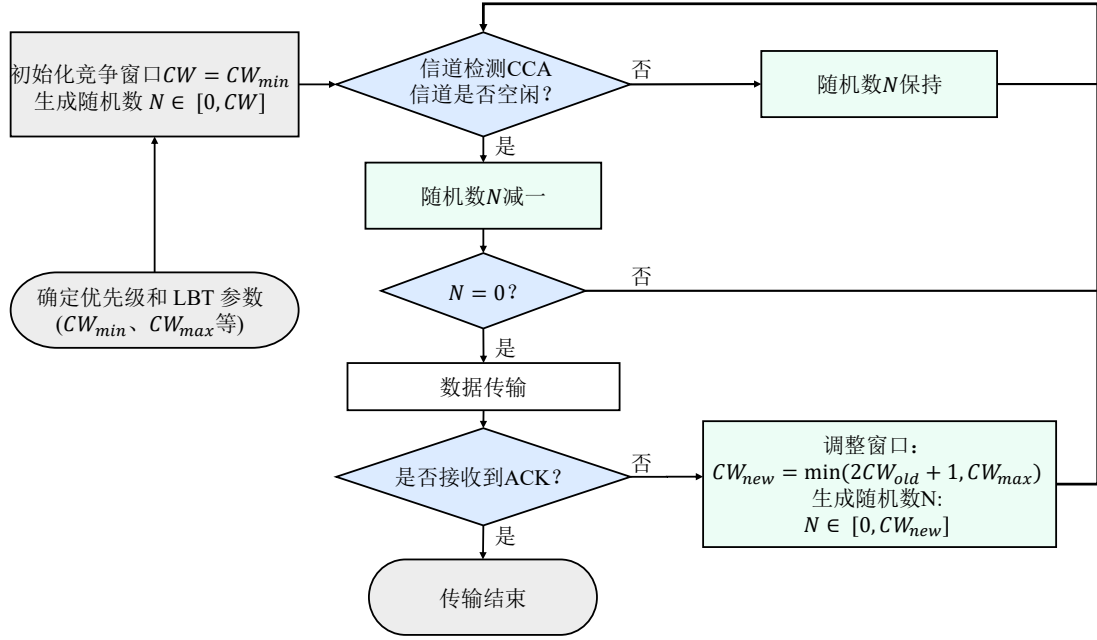
图 2-3 NR-U 中基于 LBT 的信道接入流程
