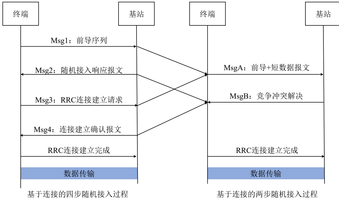
图 2-1 5G NR 两步/四步竞争式随机接入流程示意图
