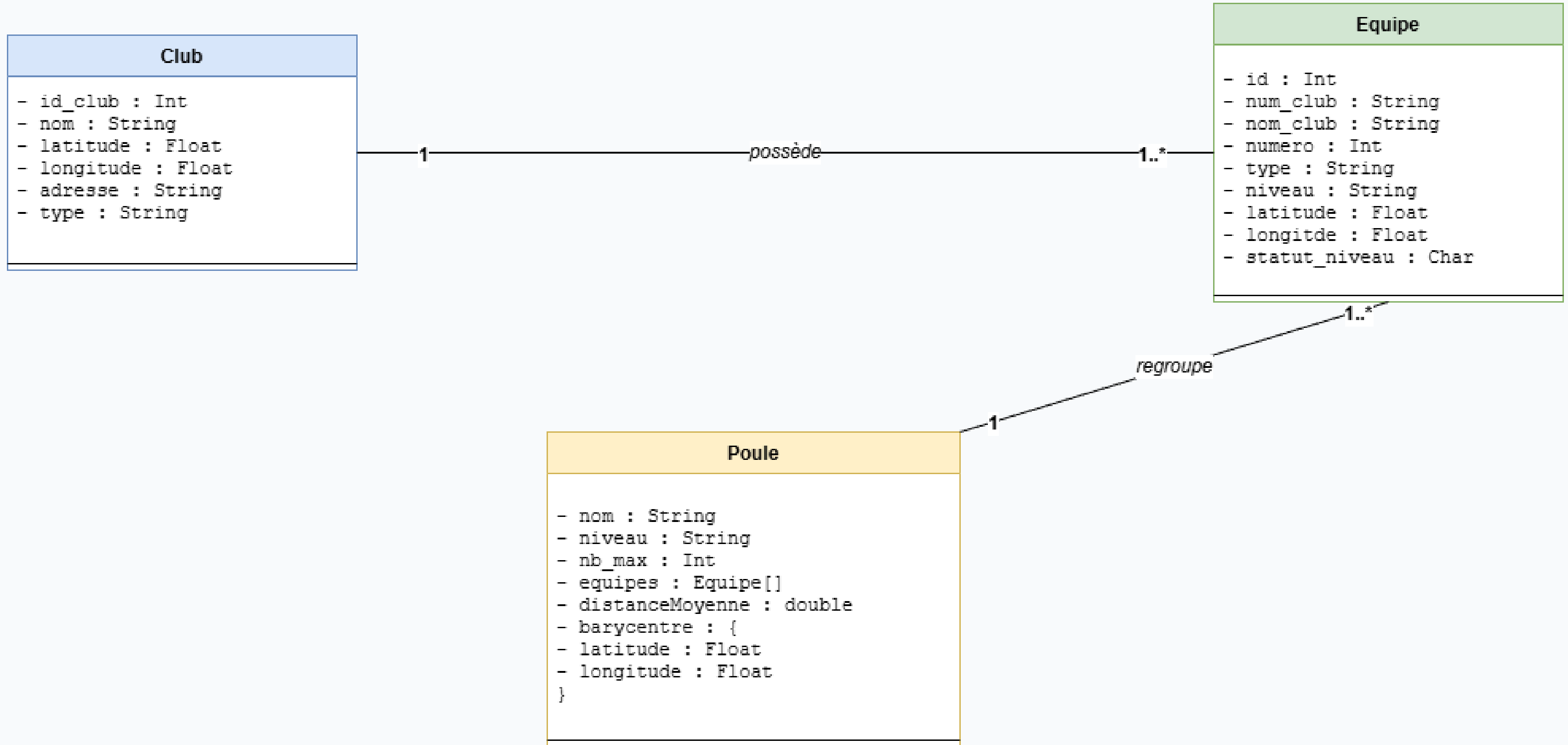
Diagramme de classes UML
