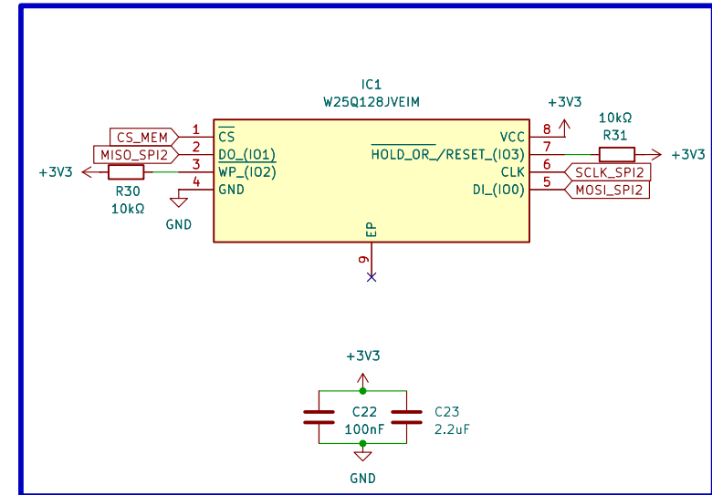
FLASH 1
