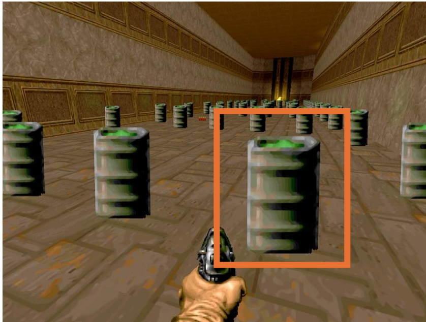
Doom
