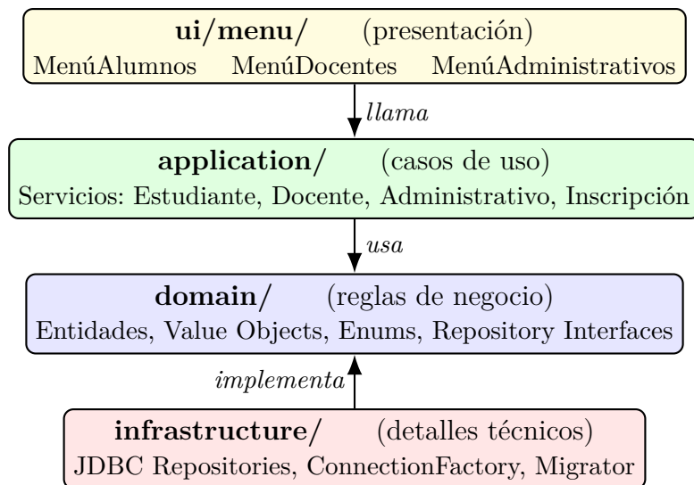
Figura 2: Las cuatro capas del sistema. La UI llama a los servicios de aplicación; éstos usan el dominio (entidades + reglas); la infraestructura implementa las interfaces que el dominio declara. La capa de dominio no conoce nada por debajo de ella.
