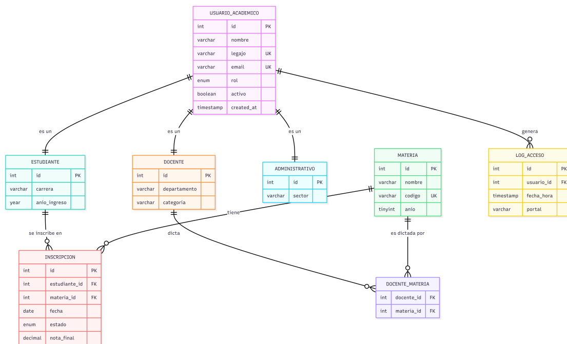
Figura 3: Diagrama UML de las entidades del dominio.
