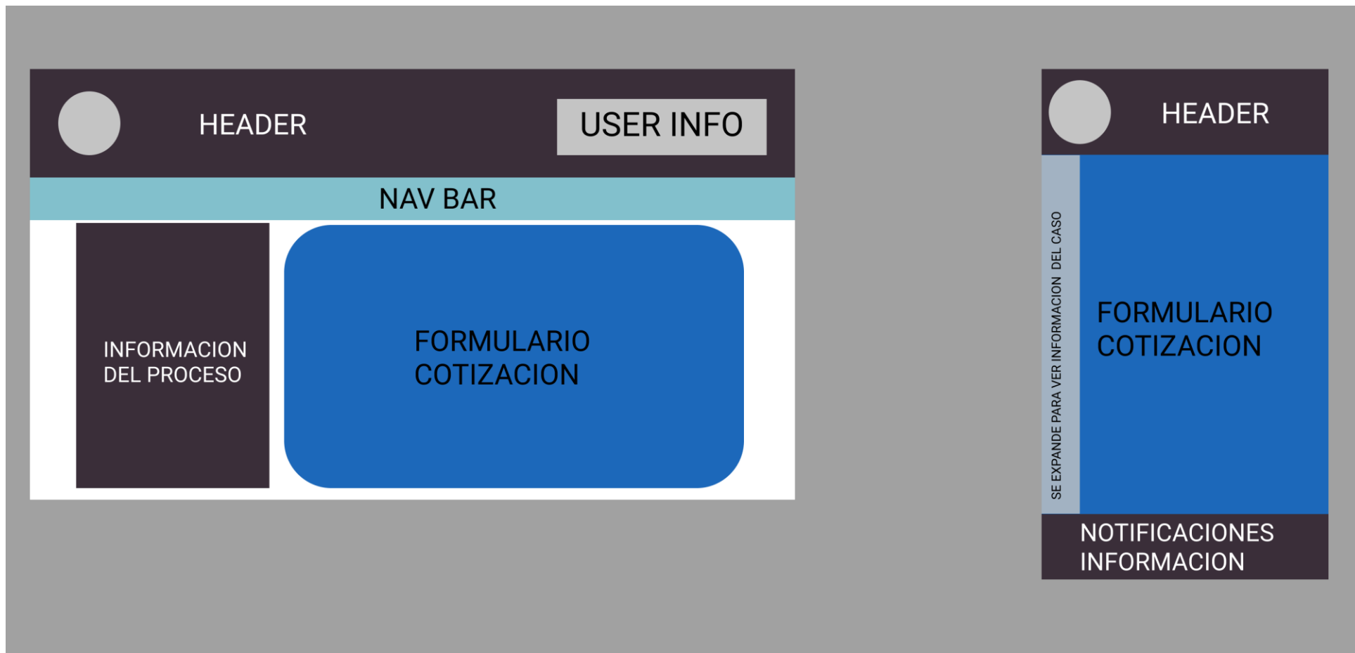
FIGURA6: COTIZACION ADMIN
