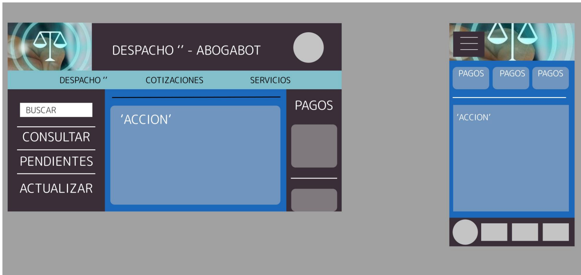
FIGURA 7: PROCESOS ADMIN
