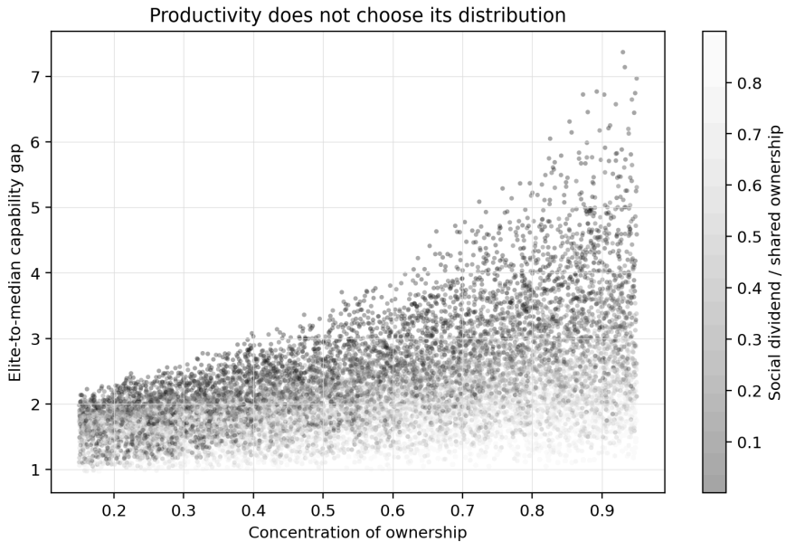
Rys. 4. Przykładowe wyjście z modelu zdolności-gap. Wyższa produktywność może współistnieć z poszerzeniem separacji między elitą a medianą efektywnej zdolności, gdy własność pozostaje skoncentrowana.
