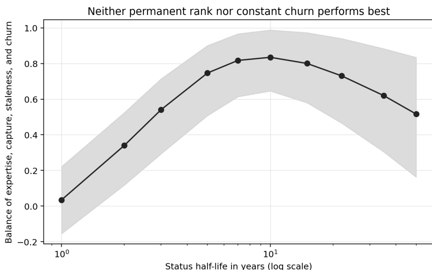
Rysunek 10. Przykładowe wyjście ze zmiany stanu w połowie życia. W modelu nie radzi sobie ani stała ranga, ani stały churn. Szczyt jest ilustracyjny i nie powinien być kopiowany jako uniwersalna długość terminu.
