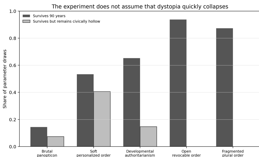
Rys. 5. Przykładowy wynik z eksperymentu nadzoru. Modelka nie zakłada, że dystopia szybko się załamuje. Miękkie i rozwojowe formy mogą przetrwać długie okresy, choć przeżycie nie jest tym samym, co głęboka stabilność.
