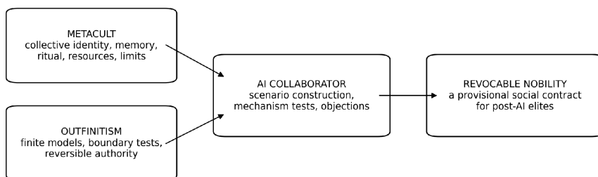
Rys. 1. Pojedynek koncepcyjny zapytania. Strzałki wskazują raczej wpływ, a nie dowód.
