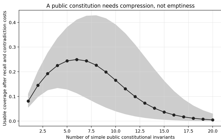
Rysunek 12. Przykładowe wyjście z zaniżania niezmiennego. W wybranym modelu dodanie małego konstytucyjnego rdzenia poprawia użyteczny zasięg; dalsze dodawanie ostatecznie traci więcej dzięki przeciążeniu poznawczemu niż zyskuje dzięki formalnej kompletności.
