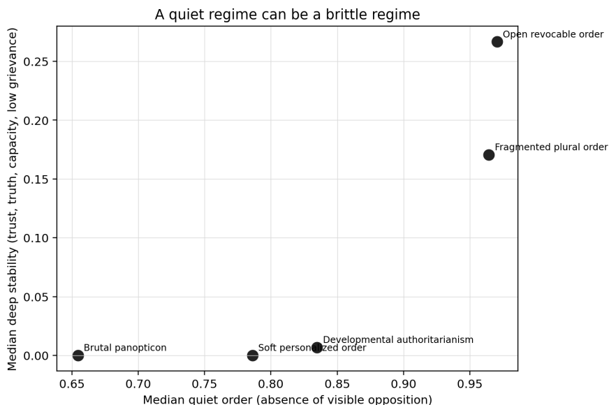
Rys. 6. Cichy porządek i głęboka stabilność rozchodzą się w modelu. Reżim może tłumić widoczny sprzeciw, tracąc jednocześnie zaufanie, jakość prawdy i zdolność korygującą.
