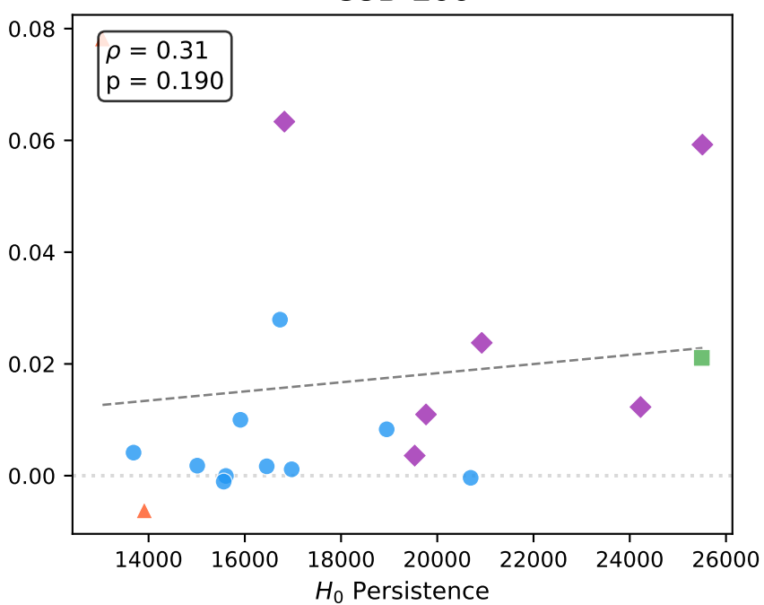
CUB-200
