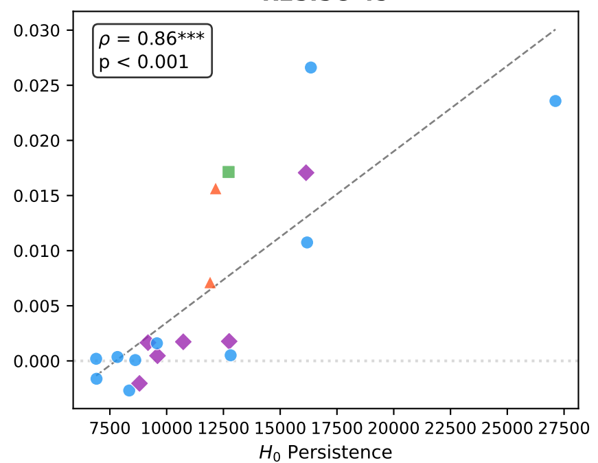
RESISC-45
