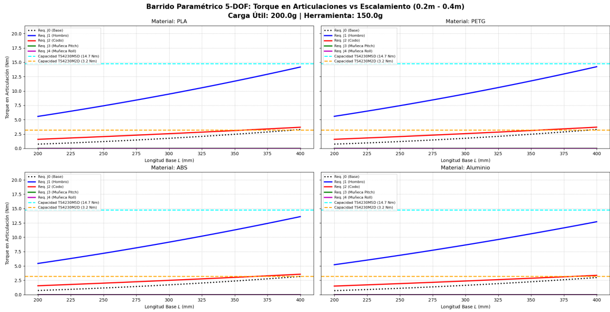
Figura 5: Barrido paramétrico (5-DOF): Requerimiento de torque incluyendo el eje de rotación de muñeca.
