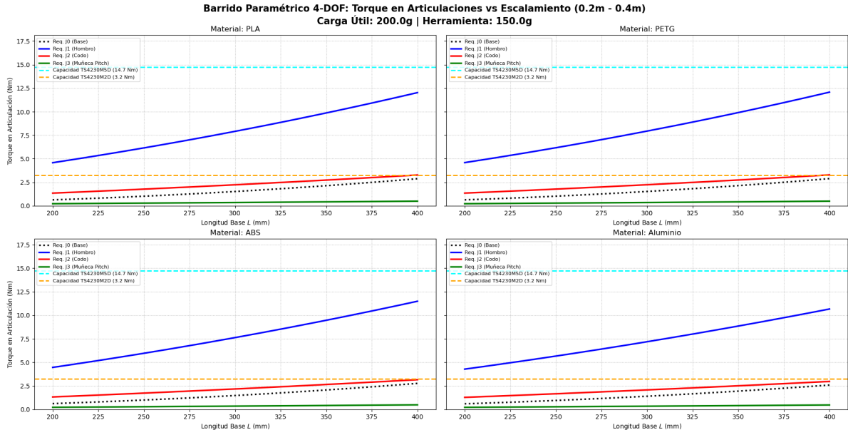
Figura 4: Barrido paramétrico (4-DOF): Requerimiento de torque en articulaciones.
