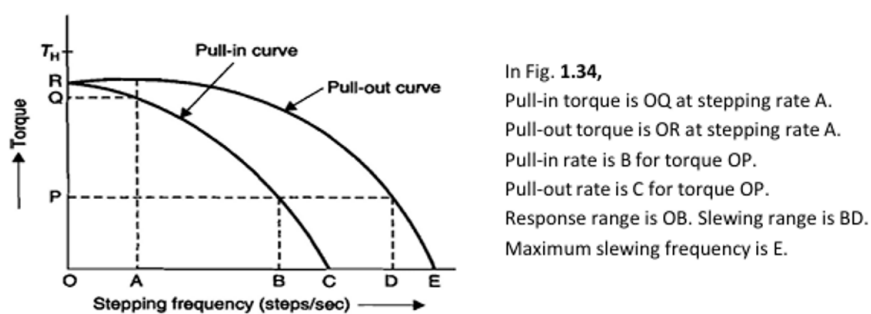
Figura 1: Curvas características de par dinámico frente a la frecuencia de pasos.
