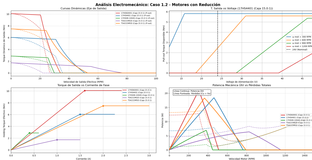
Figura 3: Curvas dinámicas (Pull-out y Pull-in) y balance de potencias.
