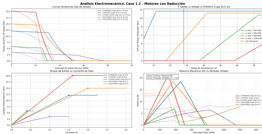
Figura 2: Curvas dinámicas (Pull-out y Pull-in) y balance de potencias.
