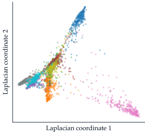
a MNIST
