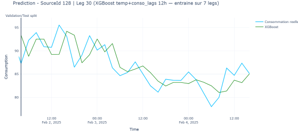
FIGURE 20 – SourceId 128, entraînement poolé sur 7 legs
