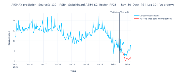
FIGURE 4 – Source 132 — ordre (0,0) : trajectoire lisse pilotée par la seule température, incapable de suivre les oscillations rapides de la consommation réelle.
