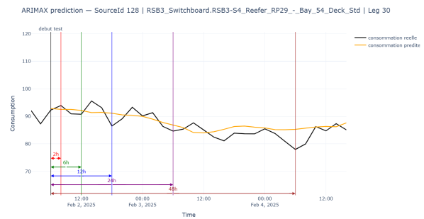
FIGURE 7 – Source 128 — trajectoire prédite quasiment superposée à la réalité sur tous les horizons, RMSE relatif \leq 4,3 %.
