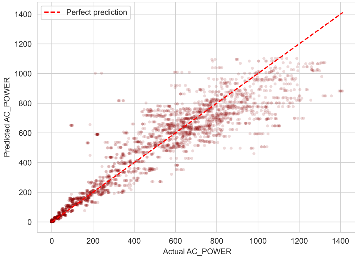
XGBoost: Actual vs Predicted (Test Set)
