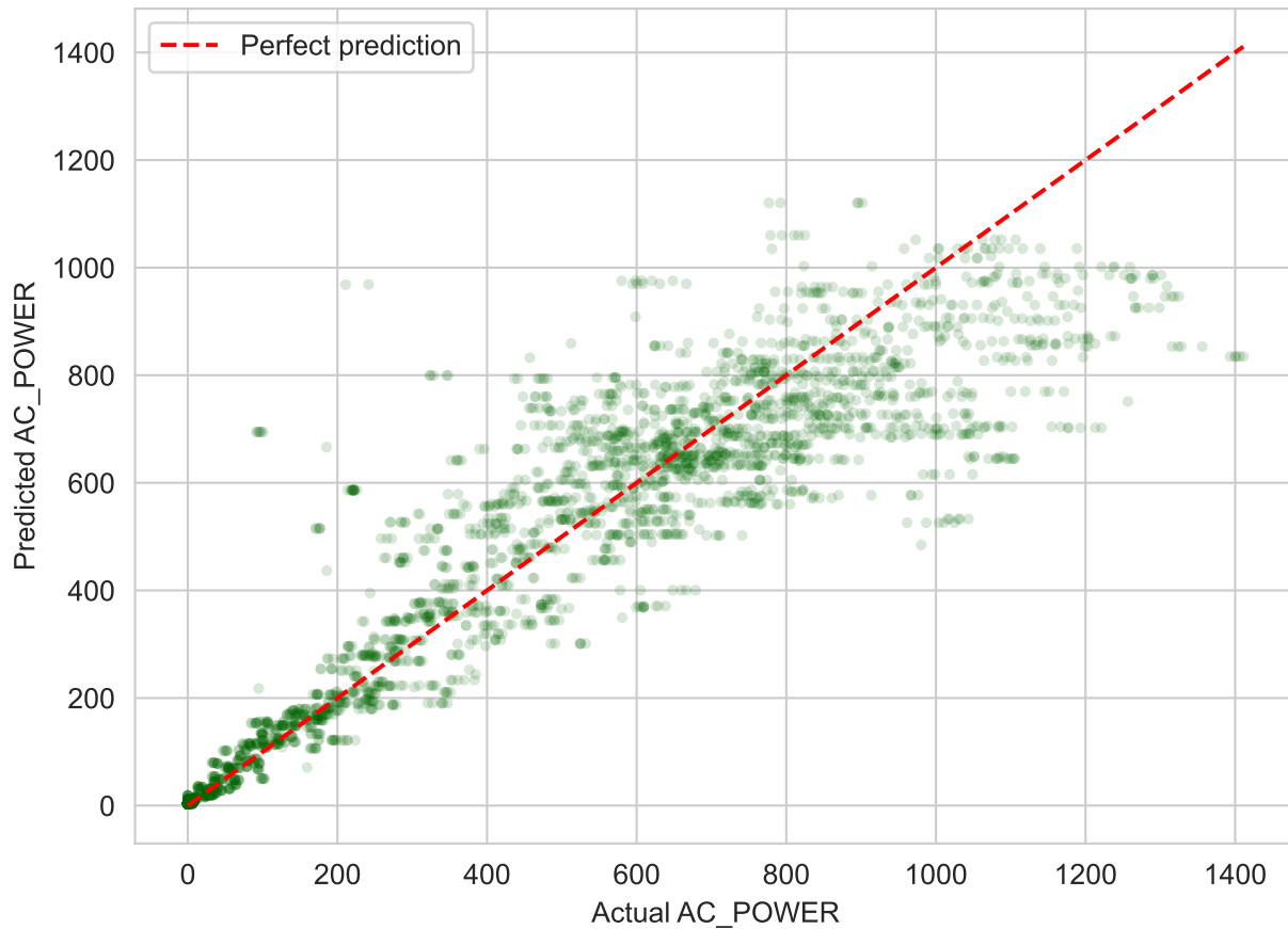
LightGBM: Actual vs Predicted (Test Set)
