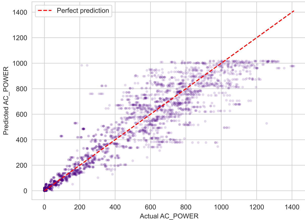
LSTM: Actual vs Predicted (Test Set)
