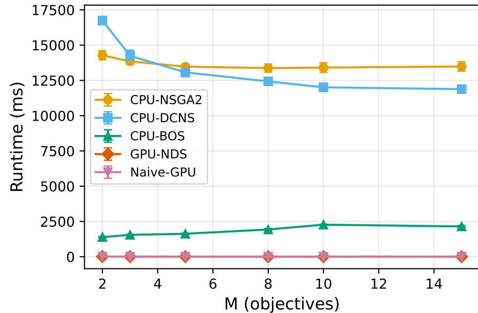
DTLZ2
