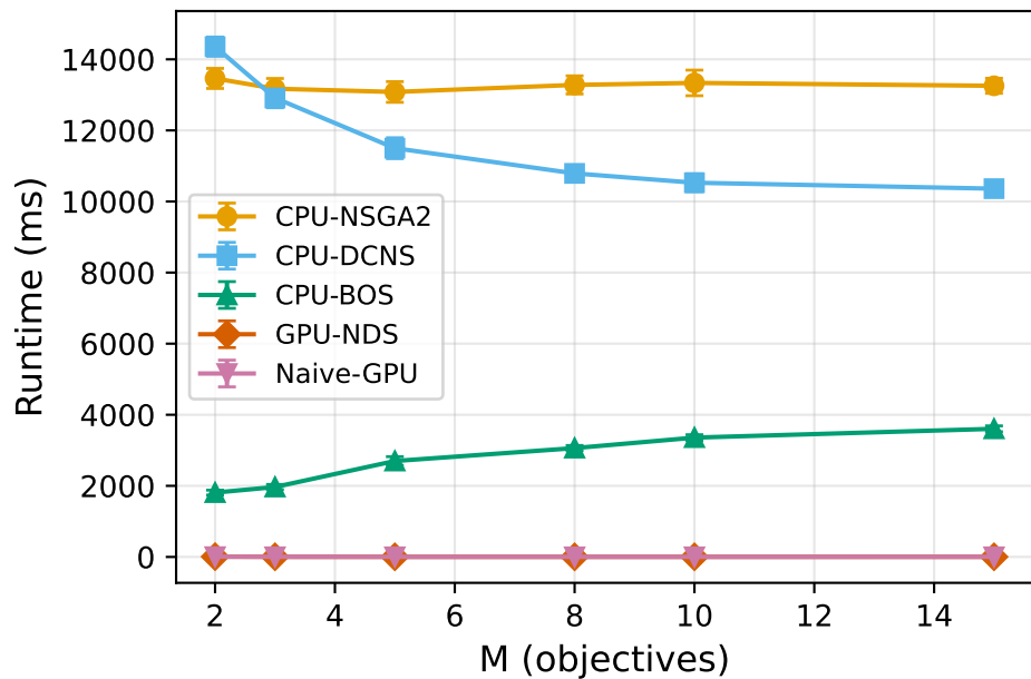
DTLZ6
