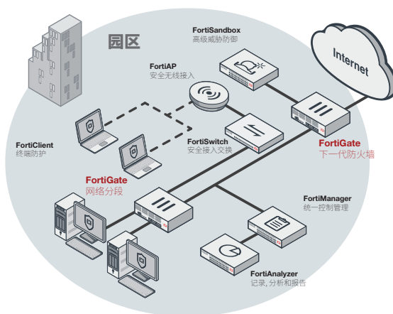
FortiGate 1500D 在园区网络中的部署 (NGFW, 基于意图的网络分段)
