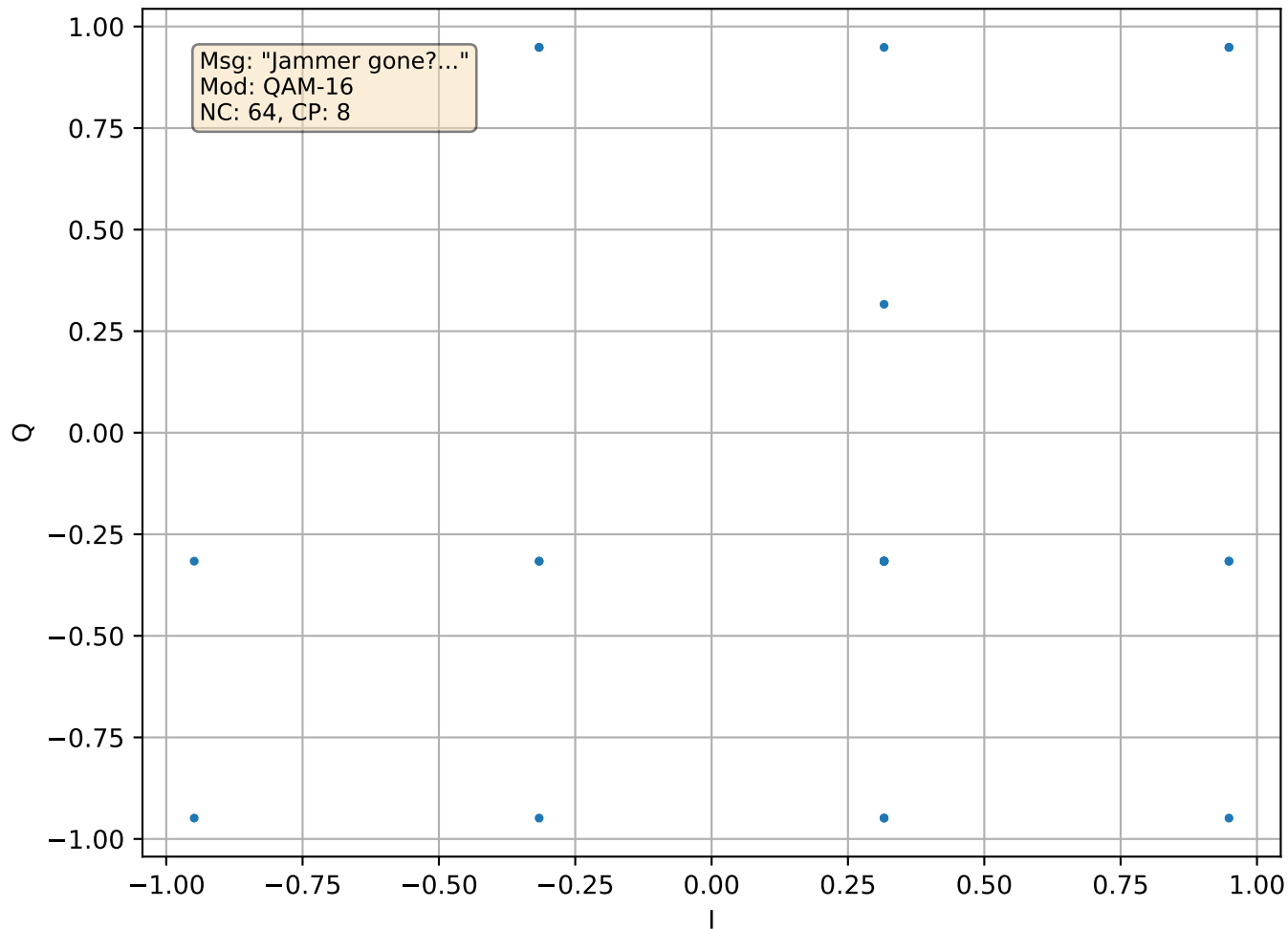
[MSG 15] R2 Constellation
