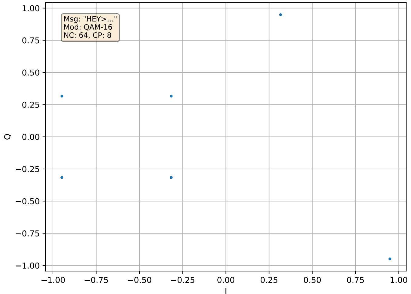
[MSG 5] R2 Constellation
