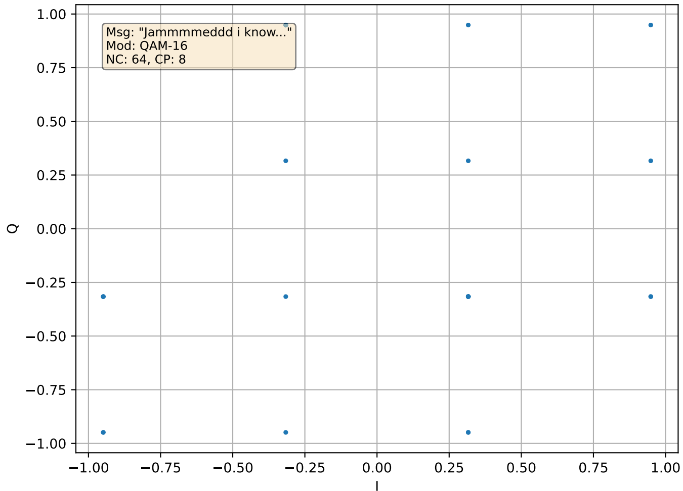
[MSG 7] R2 Constellation
