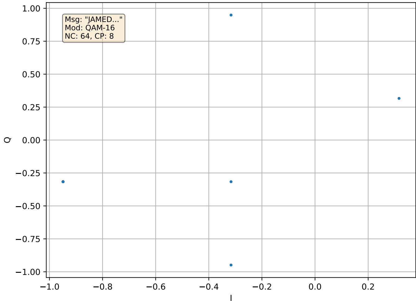
[MSG 6] R2 Constellation
