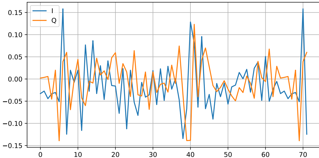
[MSG 7] R2 OFDM
