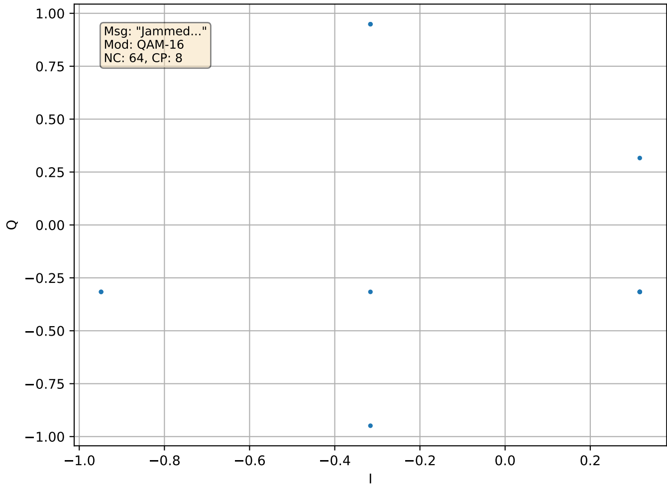
[MSG 8] R2 Constellation
