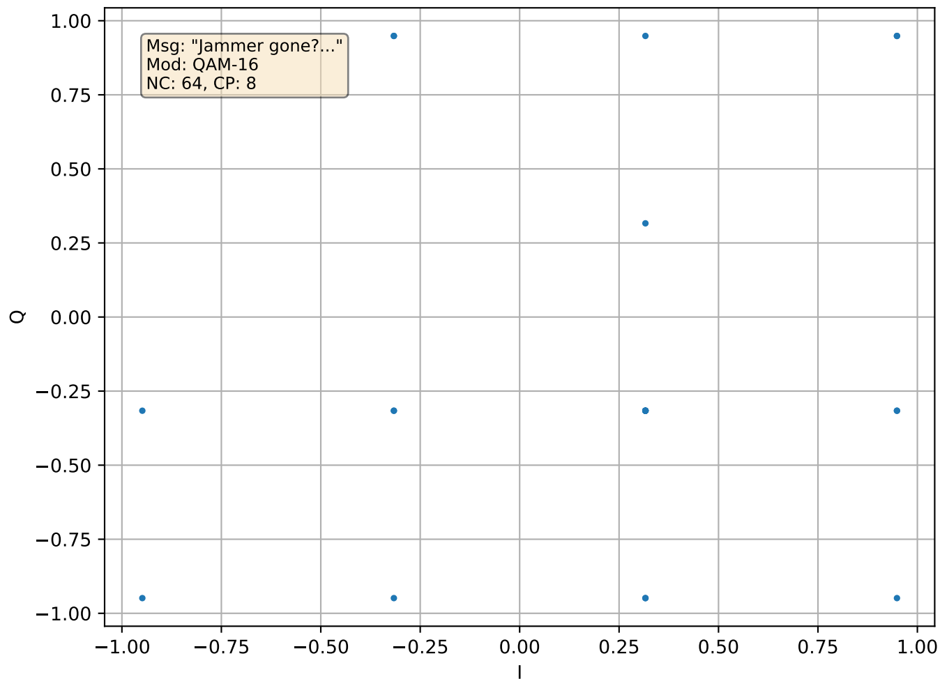
[MSG 17] R2 Constellation
