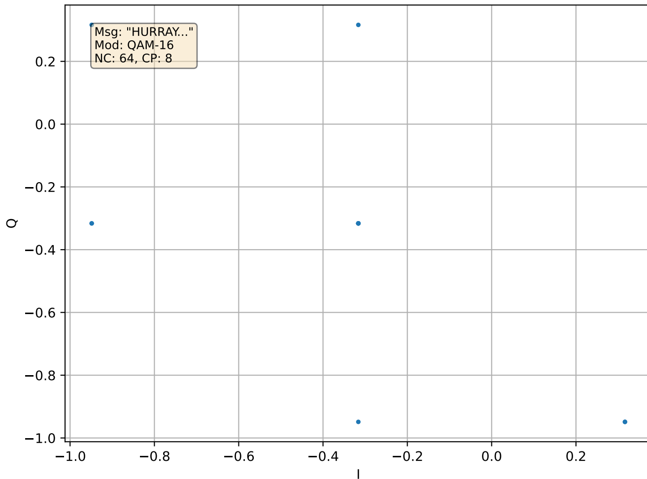
[MSG 2] R2 Constellation
