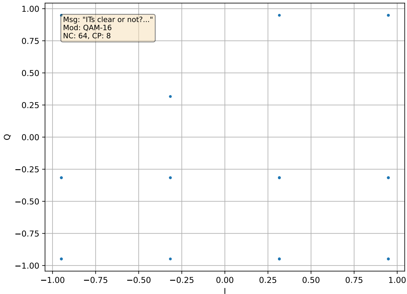
[MSG 11] R2 Constellation
