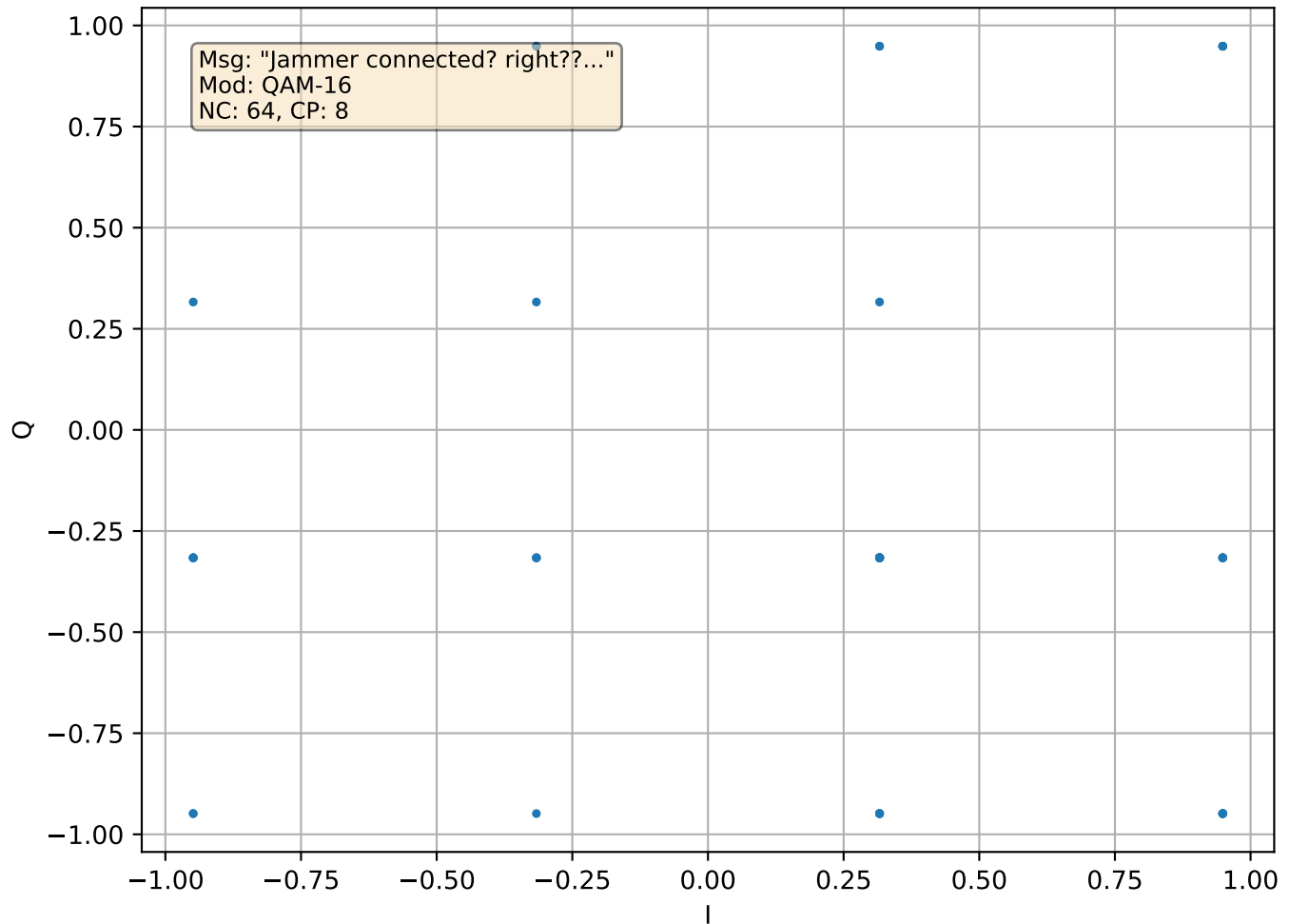
[MSG 4] R2 Constellation
