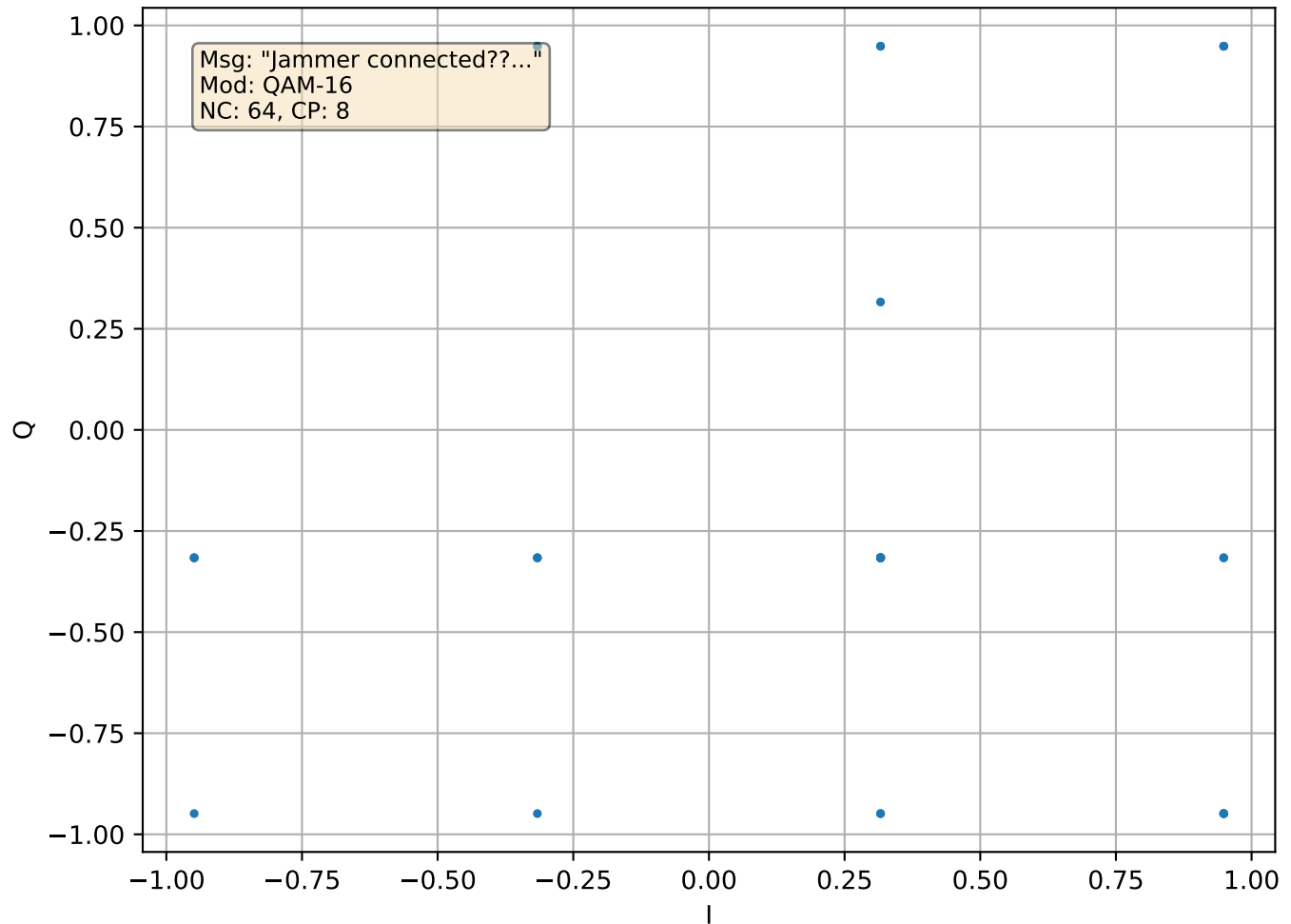
[MSG 3] R2 Constellation
