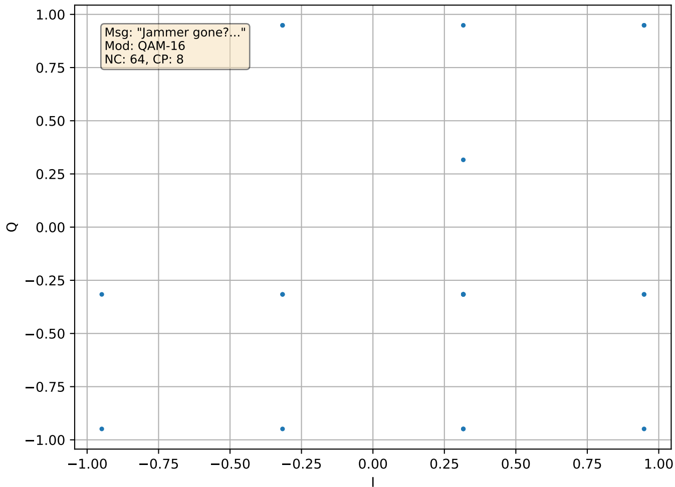
[MSG 16] R2 Constellation
