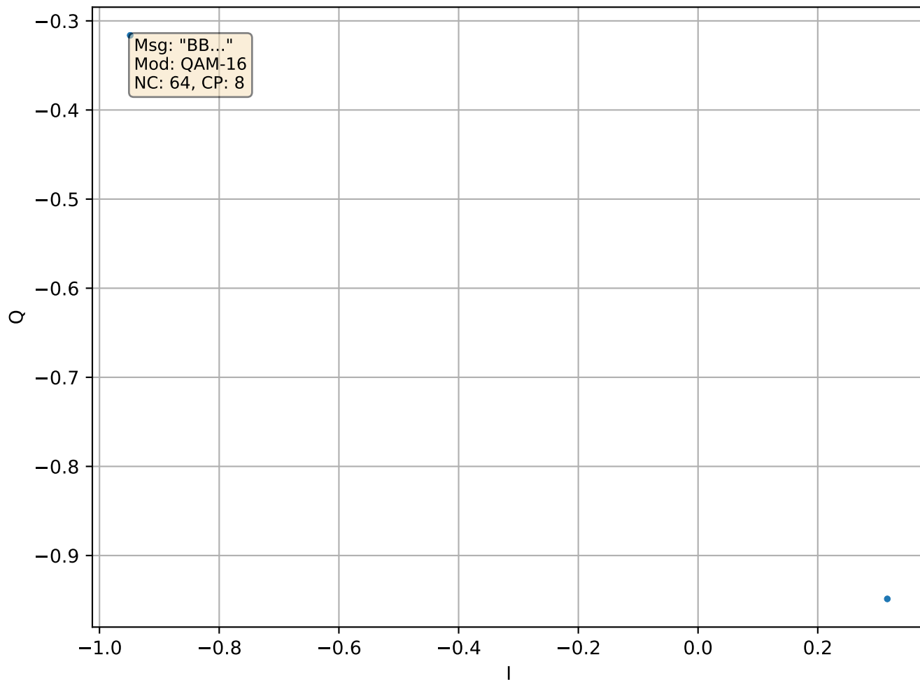
[MSG 12] R2 Constellation
