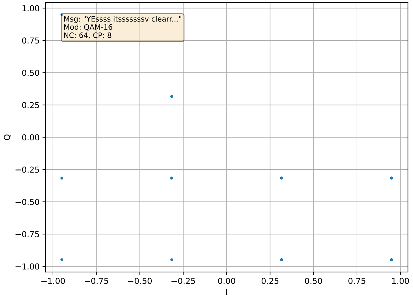
[MSG 1] R2 Constellation
