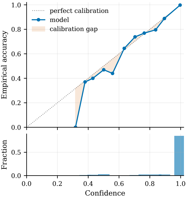
GB-META - edge_iiotset (ECE = 0.0051)
