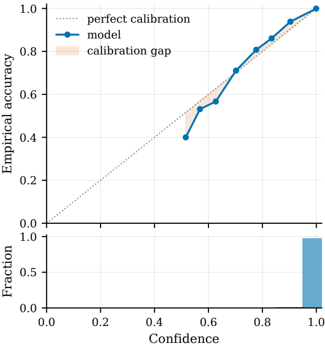
GB-META - nslkdd (ECE = 0.0009)
