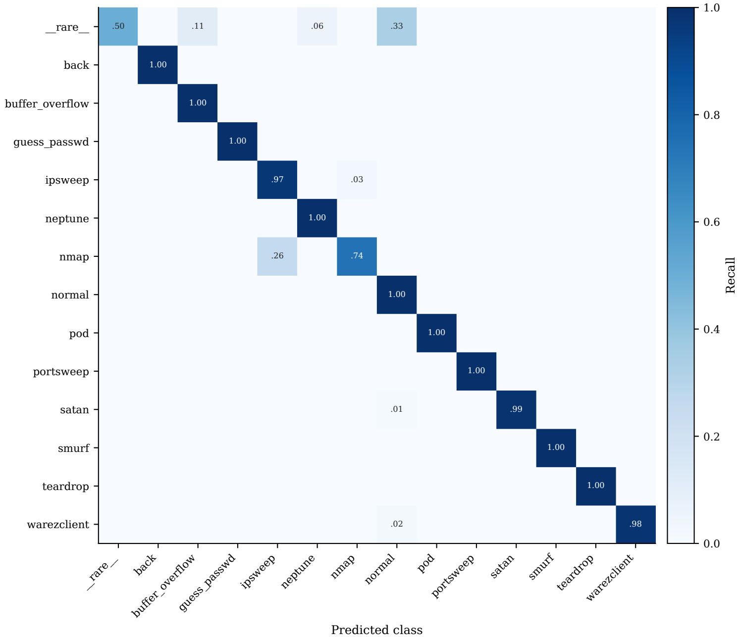
GB-META - nslkdd
