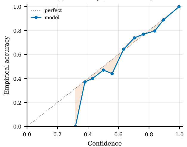
(d) Reliability (ECE = 0.0051)
