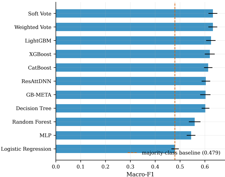
unsw_nb15
