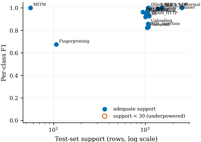
Per-class F1 vs support - edge iiotsset
