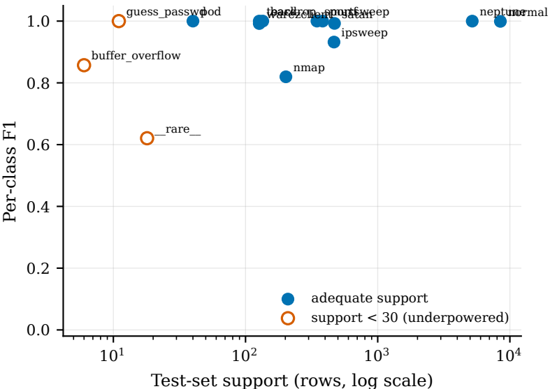
Per-class F1 vs support - nslkdd
