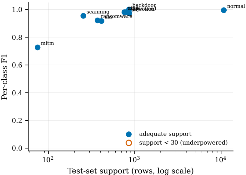
Per-class F1 vs support - ton_iot
